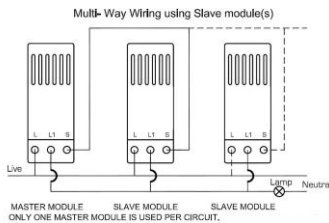
Wiring
