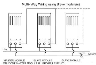
Wiring
